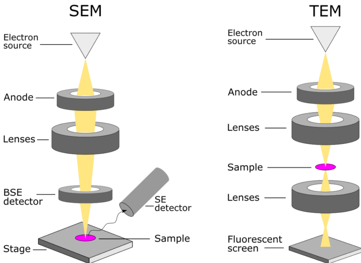
Work principle of EM
